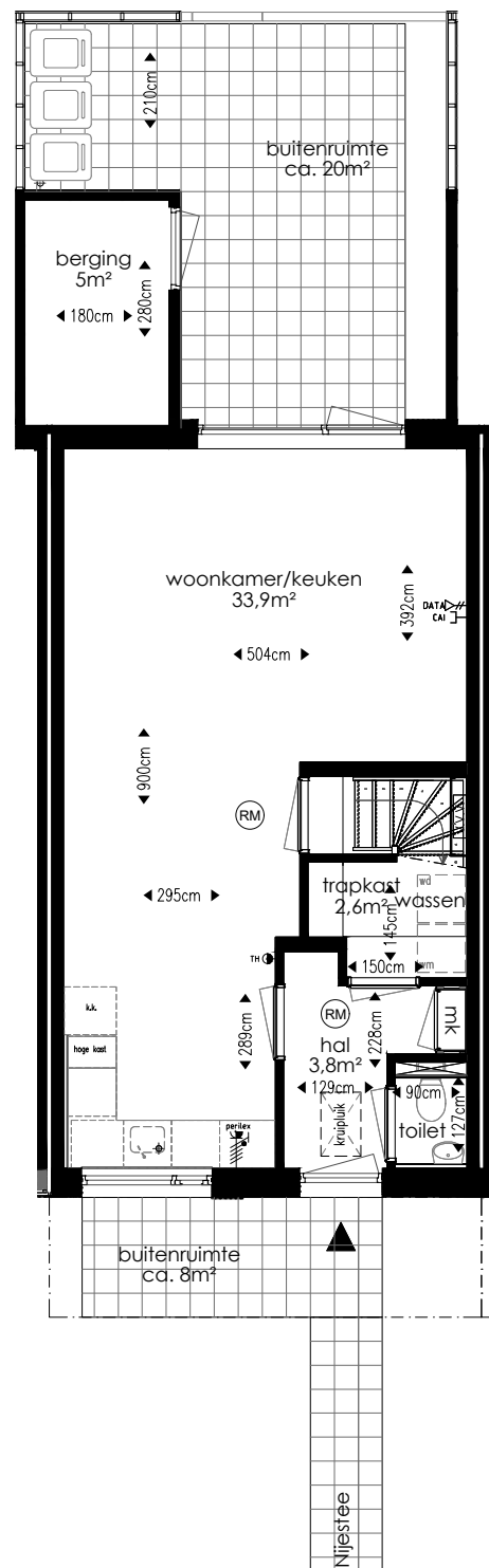
Begane grond
